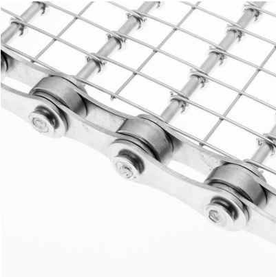
Banda metálica de malla gancho con varilla electrosoldada y cadena lateral (CMG-VE)
